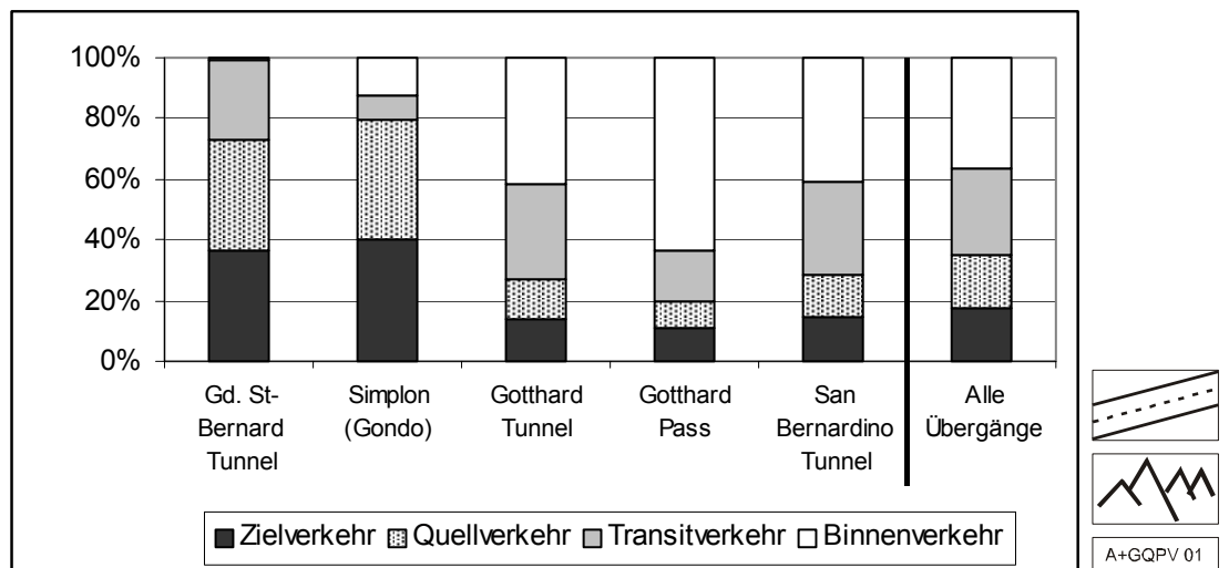
Abbildung 13: Anteile der Verkehrsarten der Personenwagen im alpenquerenden Verkehr 2001
