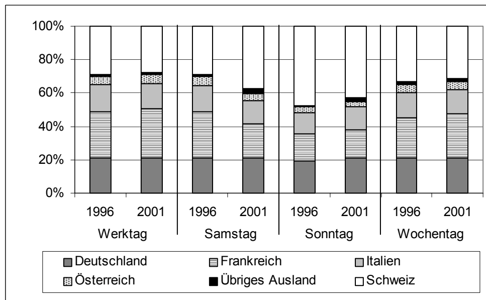
Abbildung 27: Vergleich der Immatrikulationsanteile der einreisenden Personenwagen 1996/2001 im grenzquerenden Verkehr
