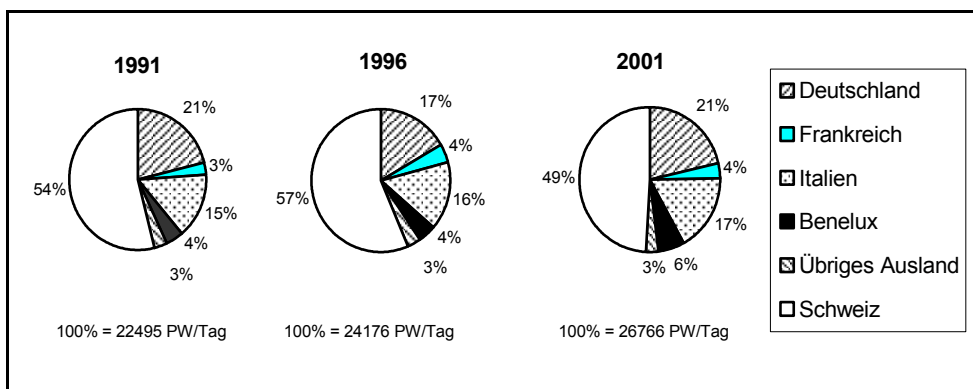
Abbildung 7: Vergleich der Immatrikulationsanteile der Personenwagen 1991/1996/2001 im alpenquerenden Verkehr
