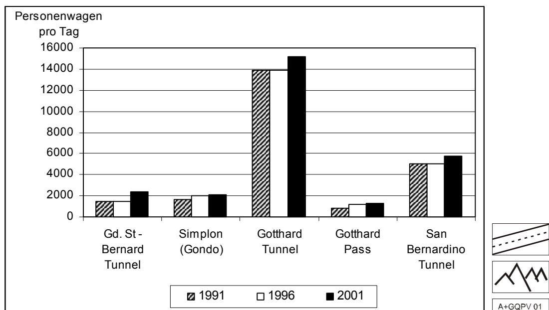
Abbildung 3: Personenwagen pro Alpenübergang 1991/1996/2001
