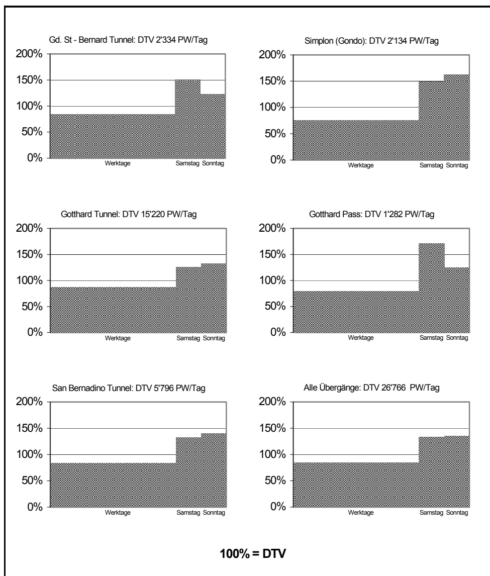
Abbildung 5: Verteilung der Personenwagen 2001 über die Wochentage (ohne Unterscheidung der Werktag) im alpenquerenden Verkehr
